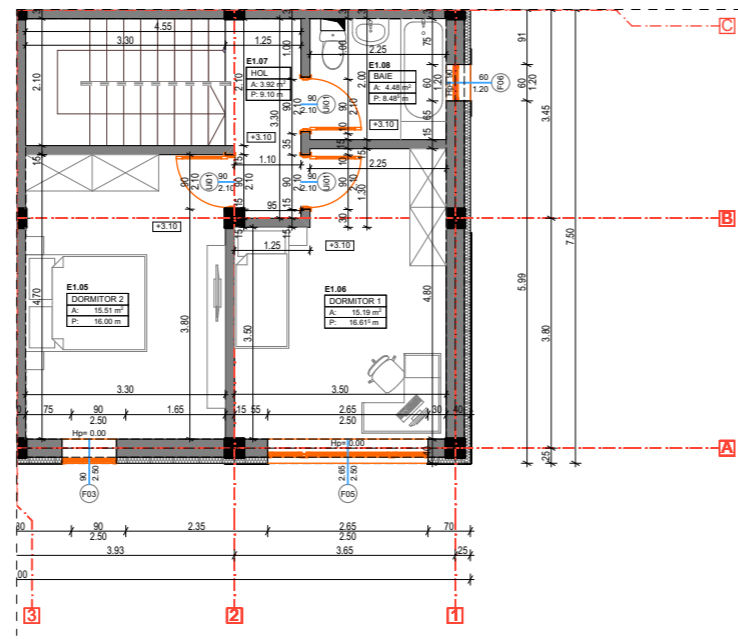
PLAN ETAJ
