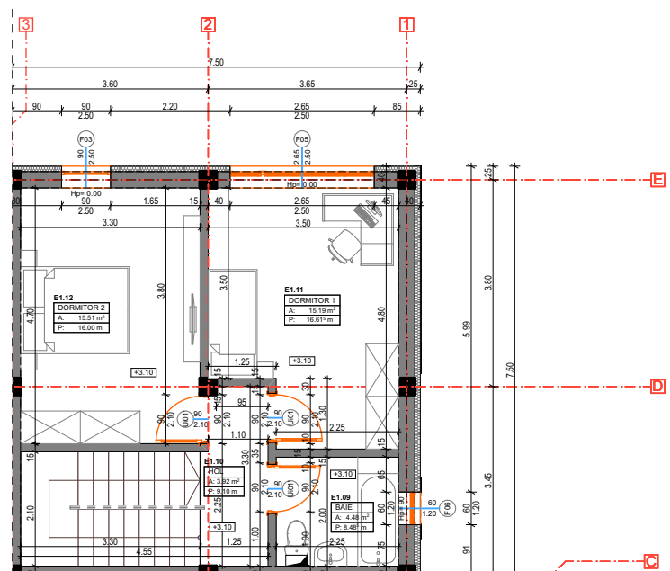
PLAN ETAJ
