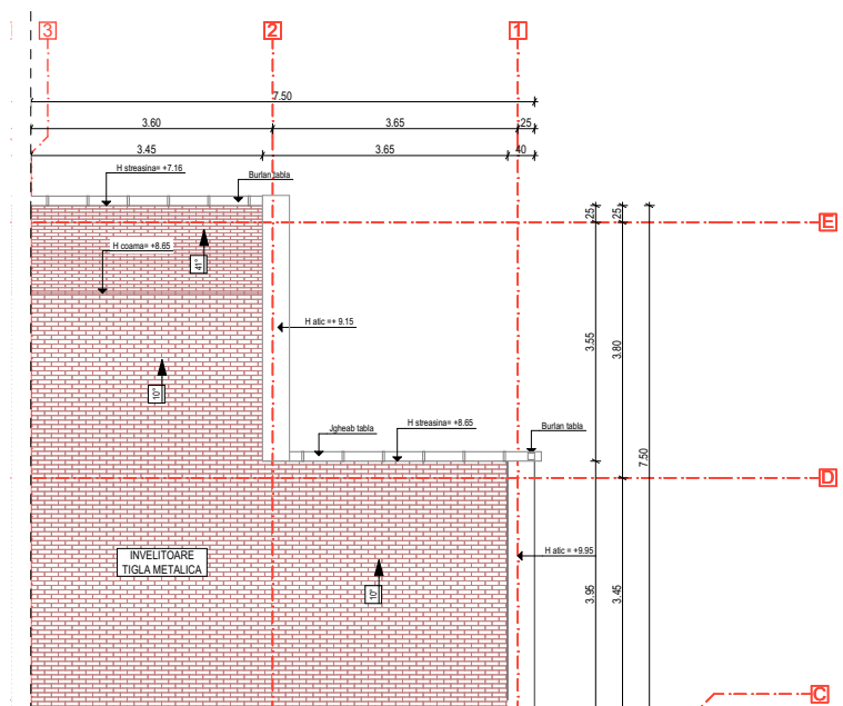
PLAN INVELITOARE
