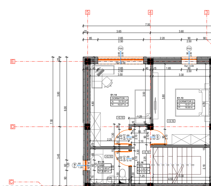
PLAN ETAJ
