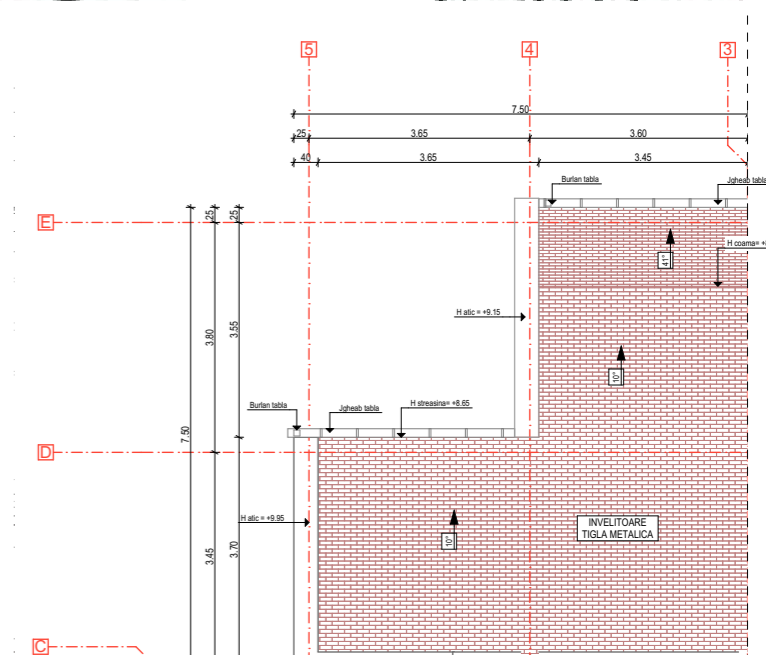
PLAN INVELITOARE
